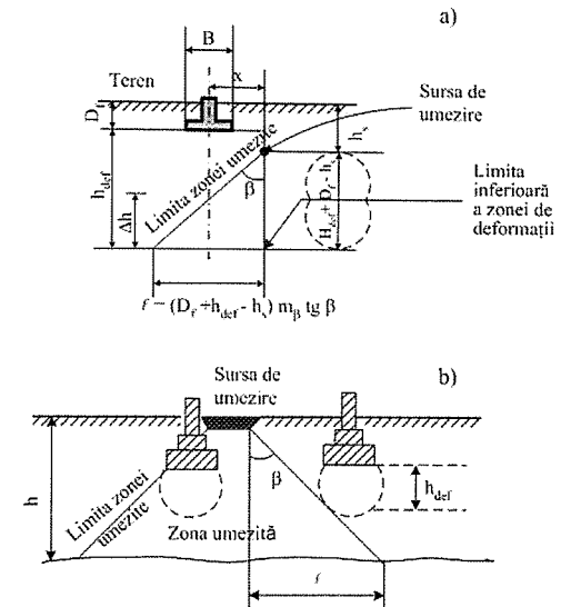
Fig. A5.2. Scheme pentru calculul tasărilor și diferențelor de tasare la umezirea PSU: a) Schema pentru stabilirea zonei inferioare de tasare suplimentară \Delta h , sub axa verticală a unei fundații situată lateral față de sursa de umezire; b) Schema pentru calculul diferenței de tasare la umezire a fundațiilor, pe terenuri din grupa A
