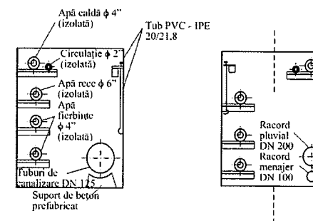
Fig. A8.2. Exemple de montare a rețelelor în canale de protecție controlabile
