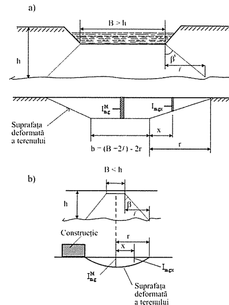
Fig. A5.3. Deformația sub greutate proprie a PSU la umezire: a) Cazul umezirii pe suprafețe mari. b) Cazul umezirii locale, pe suprafețe de dimensiuni reduse
