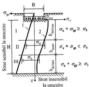
Fig. 1. Zone caracteristice în terenul de fundare alcătuit din pământuri sensibile la umezire: I - zonă deformabilă superioară; II - zonă inertă; III - zonă deformabilă inferioară; 1 - diagrama variației cu adâncimea a efortului \sigma_{gz} ; 2 - diagrama variației cu adâncimea a efortului \sigma_z
