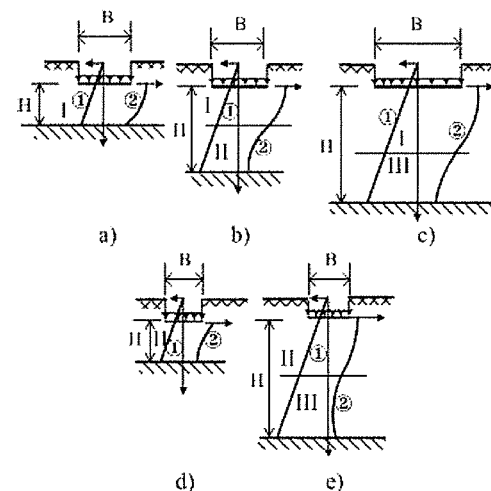
Fig. 2. Situații caracteristice pentru terenul de fundare alcătuit din pământuri sensibile la umezire: I - zonă deformabilă superioară; II - zonă inertă; III - zonă deformabilă inferioară; 1 - diagrama variației cu adâncimea a efortului \sigma_{gz} ; 2 - diagrama variației cu adâncimea a efortului \sigma_z
