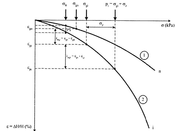
Fig. A5.1. Curbe de compresiune medii pentru probe netulburate, cu umiditatea naturală (curba 1) și inundate inițial (curba 2)
