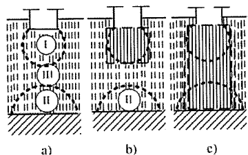
Fig. 4. Variante de fundare pe un teren din grupa B
