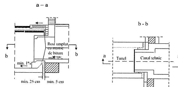
Fig. A8.3. Asigurarea continuității protecțiilor din clădire la exterior (exemple) În subsol, obligatoriu conductele se vor monta aparent.
